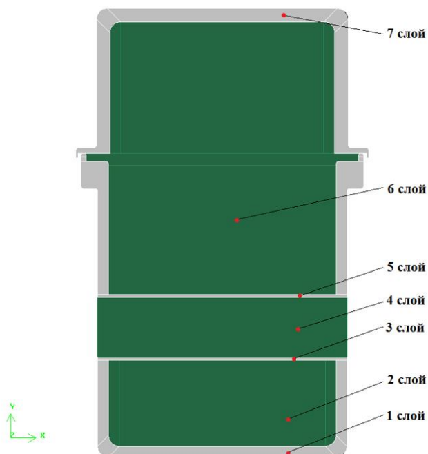
Рис. 2. Семислойная конструкция термощафа
