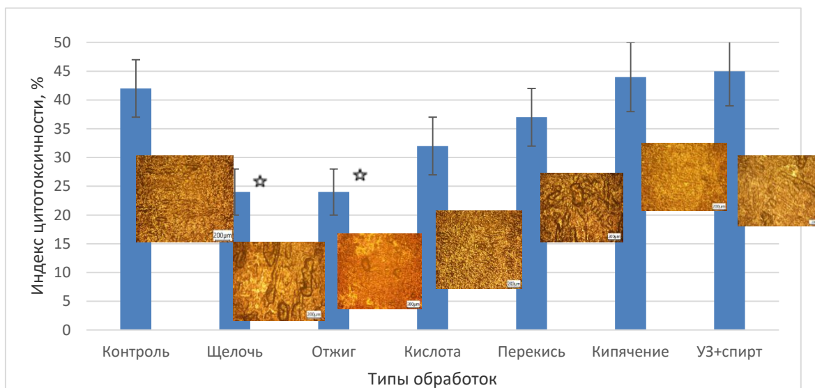
Рис. 1. – Индекс цитостатического влияния образцов из никелида титана марки TN-10, после различных методов стерилизации и модификации поверхности, на клетки линии 3Т3
