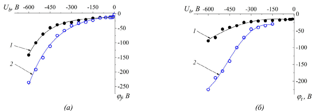
Рис. 3 – Плавающий потенциал \varphi_f зонда (а) и потенциал диэлектрических мишеней \varphi_i (б) как функции потенциала U_b на пластине: 1 – алюмооксидная керамика; 2 – кварц. Давление 2 Па, ток пучка 2 мА, энергия пучка 3 кэВ
