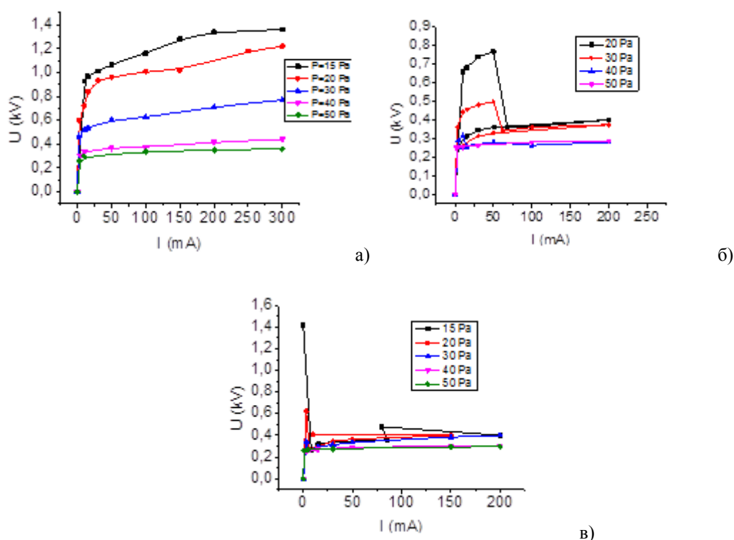
Рис.2. Вольтамперные характеристика разряда при различных значениях давления газа (Ar). Значения диаметров отверстий, d: а) 0,6мм; б) 2,5мм; в) 4 мм
