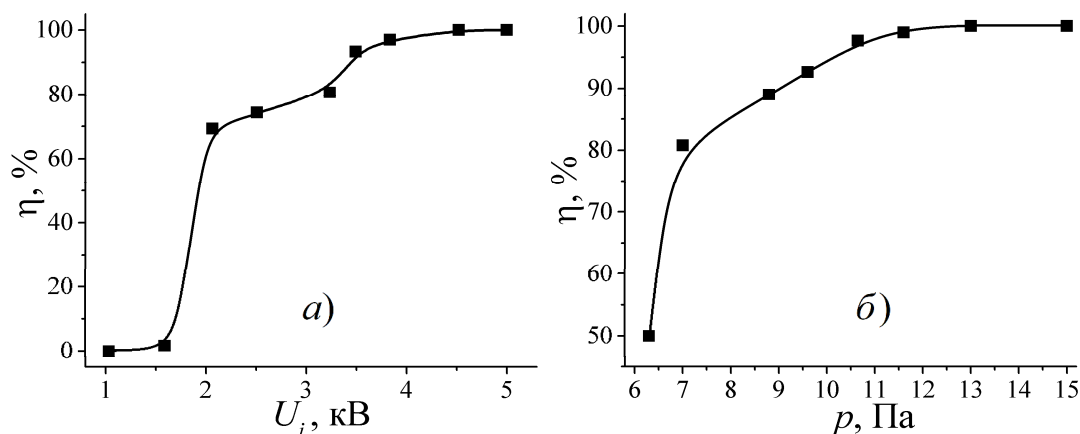
Рис 2. Зависимости вероятности \eta инициирования контрагированного дугового разряда от амплитуды U_i поджигающего импульса при p = 8 Па (а) и от давления газа p при U_i = 2,5 В (б)
