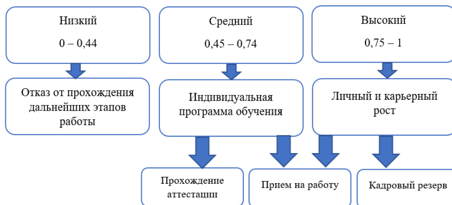
Рис. 2. Уровни благонадежности в рекомендательной системе кадровой безопасности предприятия
