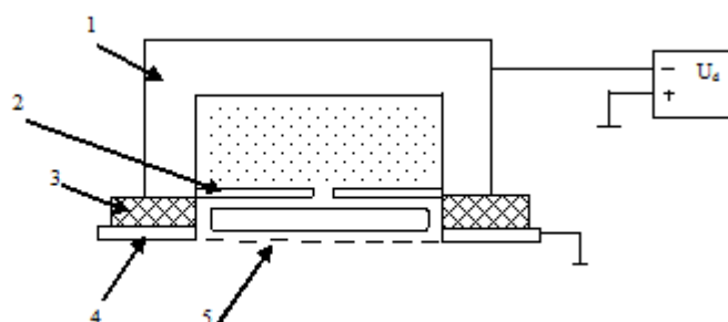
Рис.1. Схема форвакуумного плазменного источника ленточного электронного пучка 1 - Катод; 2 - металлические пластины; 3 - Изолятор; 4 - Анод; 5 - Сетка
