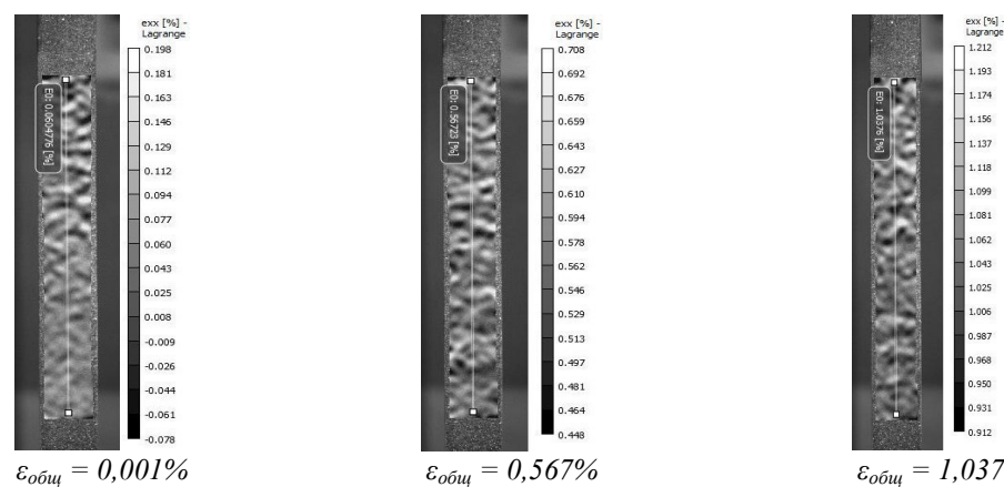
Рис. 3. Картины деформационных полей продольных относительных деформаций углекомпозиата с преднапряжением при разных значения деформации
