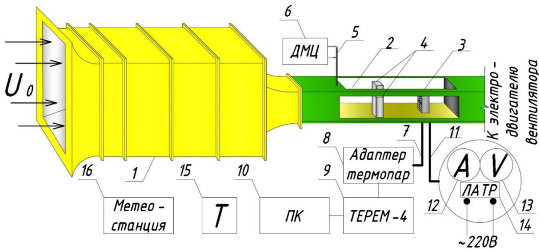
Рис. 1. Блок-схема аэродинамического стенда: 1 – диффузор аэродинамической трубы; 2 – рабочая камера; 3 – исследуемая модель; 4 – модель-препятствие; 5 – трубка Пито-Прандтля; 6 – манометр цифровой ДМЦ-01М; 7 – термопары; 8 – адаптер термопар; 9 – регистрирующий блок ТЕРЕМ-4; 10 – компьютер; 11 – силовые кабели; 12 – амперметр; 13 – вольтметр; 14 – ЛАПР; 15 – термометр; 16 – электронная метеостанция
