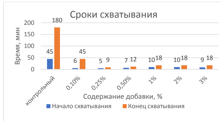
Рис. 1. Влияние добавки гидрокарбоната натрия на сроки схватывания цемента
