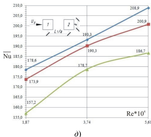
Рис. 2. Графики влияния скорости ветрового потока на средний по граням коэффициент теплообмена (через число Нуссельта Nu ) модели «2» при угле атаки \varphi=0^\circ : а) – L1/a = 1 ; б) – L1/a = 4 ; в) – L1/a = 6 ; г) – L1/a = 10 ; д) – L1/a = \infty (одиночная модель)
