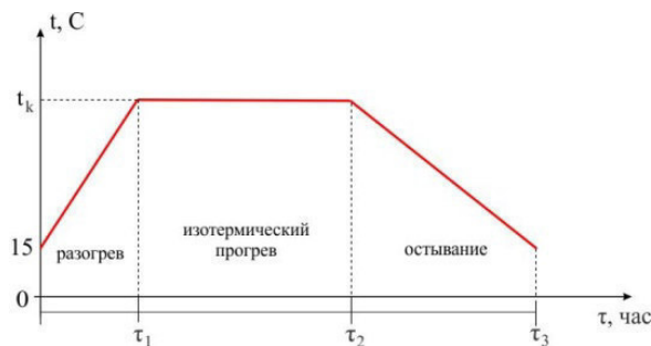
Рис. 2. Режим выдерживания бетона монолитного перекрытия с помощью греющего провода ПНСВ-1.2: \tau_1 , \tau_2 , \tau_3 – продолжительность (час) периода разогрева бетонной смеси, изотермического выдерживания и остывания бетона соответственно
