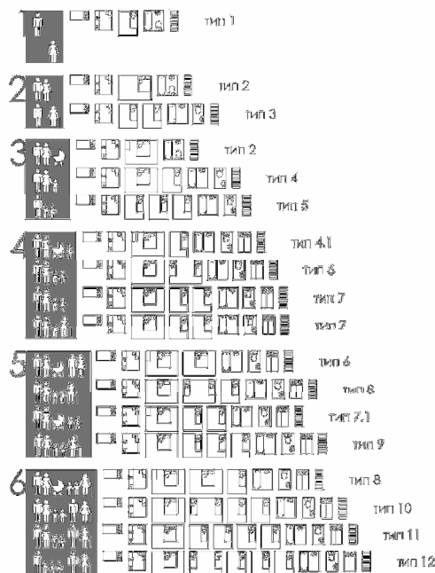
Рис. 2. Типологический ряд жилых ячеек социального типа для семей г. Томска
