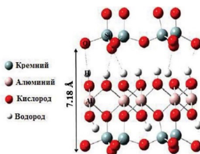
Рис. 1. Структура каолина
