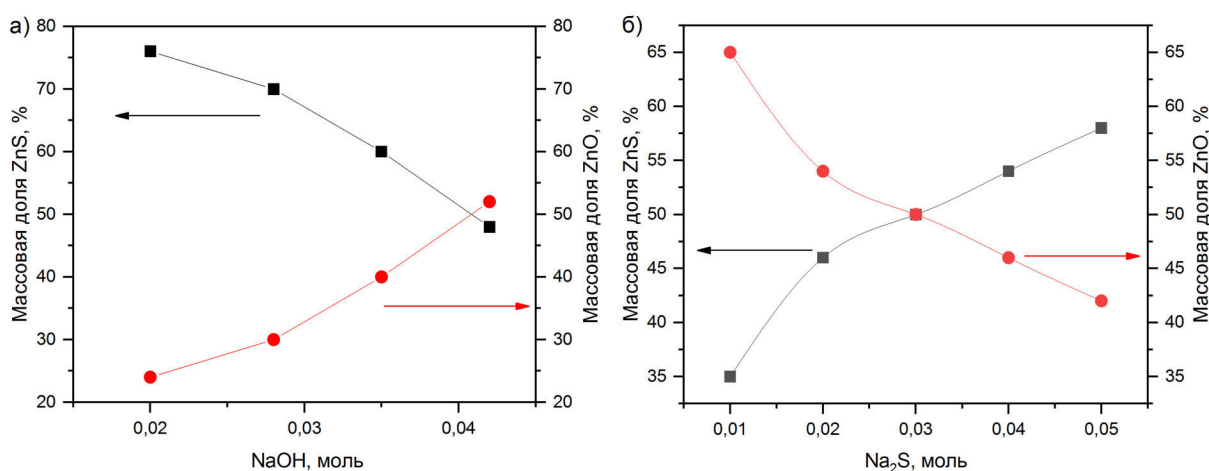
Рис. 1. Влияние количества прекурсоров, участвующих в формировании оболочки, на фазовый состав образцов на основе ZnS@ZnO (а) и ZnO@ZnS (б)
