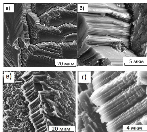
Рис. 2. Микрорельеф поверхности излома образцов монокристаллов Ni_3Ge (а, б) и Ni_3Al (в, г) в исходном состоянии, разрушенных в схеме на изгиб при комнатной температуре
