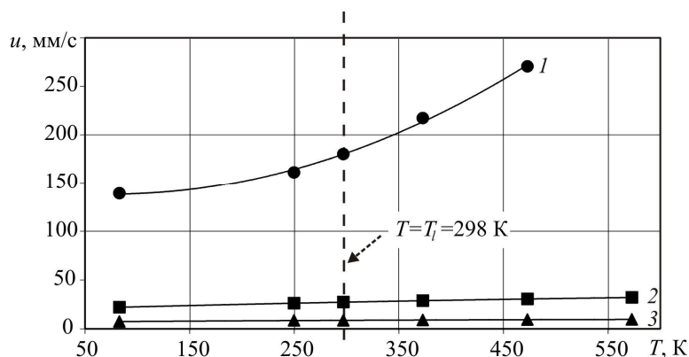
Рис. 2. Зависимость скорости частицы ( D_p = 8.7 мкм) от ее температуры в процессе гравитационного осаждения в глицерине (1); ПМС-10000 (2); ПМС-30000 (3)
