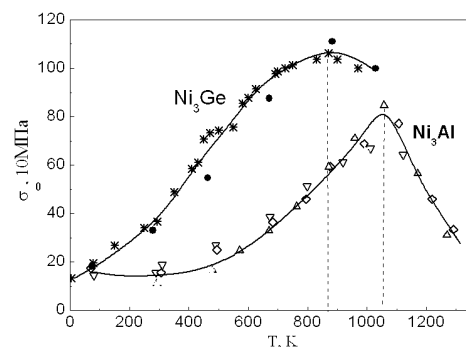
Рис. 1. Сравнение температурных зависимостей предела текучести монокристаллов сплавов Ni_3Ge и Ni_3Al ориентации [0 0 1] по данным разных авторов [1]
