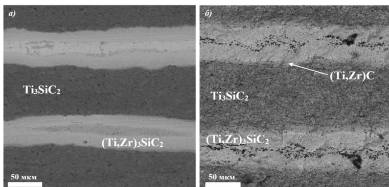
Рис.2. СЭМ изображение поверхности композита на основе системы Ti_3SiC_2/Zr , полученного при температуре 1400\text{ }^\circ\text{C} (а) и 1600\text{ }^\circ\text{C} (б) и давлении 50\text{ МПа}
