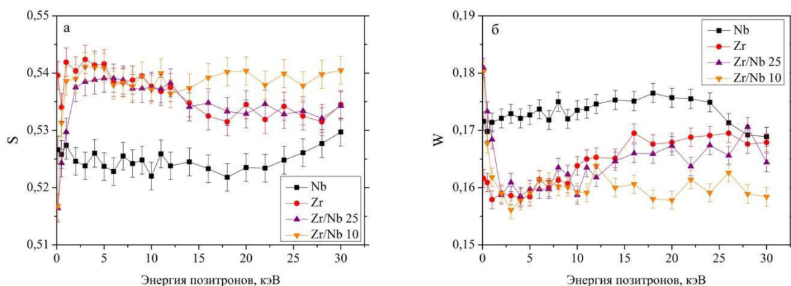
Рис. 2. График зависимости S параметра (а) и W параметра (б) от энергии позитронов для НМП Zr/Nb с толщиной индивидуальных слоев 25 \pm 2 нм и 10 \pm 1 нм, а также монослойных покрытий Zr и Nb
