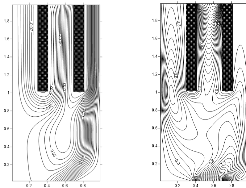
Рис. 2. Распределение изолиний функций тока (слева) и изолиний окружной составляющей вектора скорости (справа) в вихревой камере при параметрах течения R_e=20 ; R_{\omega 0}=4 ; R_{\omega 1}=4 ; R_{\omega d}=0
