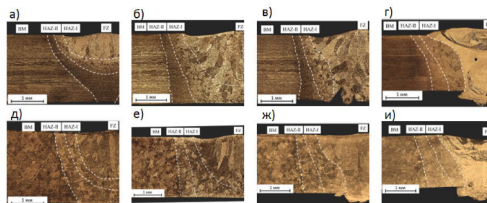
Рис. 1. Металлографические изображения поперечных шлифов проката и SLM образцов при различной силе тока: прокат: а, б, в, г – 20, 25, 30, 35 мА соответственно, SLM образец: д, е, ж, и – 20, 25, 30, 35 мА соответственно
