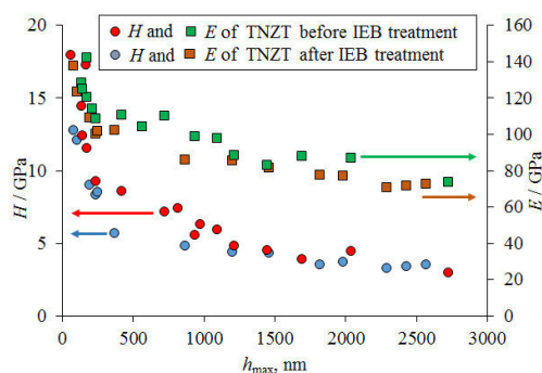
Рис. 2. График зависимости нанотвердости ( H ) и значения модуля Юнга ( E ) от глубины инденитирования ( h )
