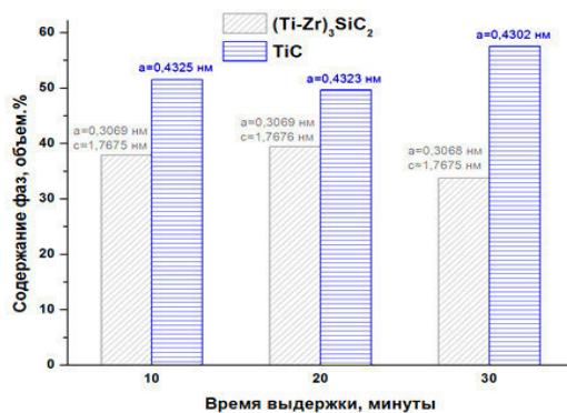
Рис. 3. Зависимость соотношения фаз для синтезируемых композитов на основе системы Ti_3SiC_2/Zr от времени спекания ( 1400\text{ }^\circ\text{C} , 50\text{ МПа} )
