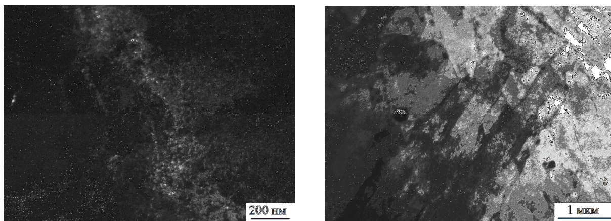
Рис. 2. Микроструктура стали ЭП-823 после ВТМО: а) темнопольное изображение в рефлексе частиц типа MX ; б) светлопольное изображение ферритно-мартенситной структуры, содержащей карбиды M_{23}C_6
