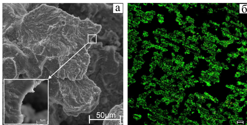
Рис. 1. РЭМ изображения поверхности разрушения TiNi (а) и конфокальная микроскопия поверхности TiNi с клетками MCF-7 (б)
