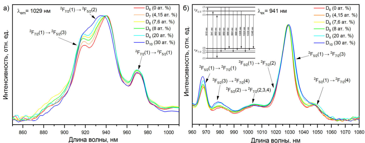
Рис. 1. Нормализованные спектры фотовозбуждения люминесценции (а) и люминесценции (б) порошков YSAG:Yb с различным содержанием скандия
