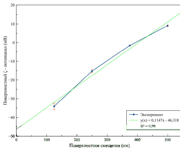
Рис. 2. График значения поверхностного ζ-потенциала обработанного, спеченного образца Al_2O_3 с 15% пористостью
