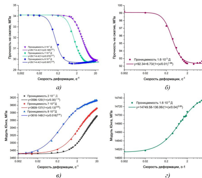
Рис. 1. Зависимости прочности на сжатие (а,б) и модуля Юнга (в,з) губчатой (а,в) и кортикальной (б,з) костной ткани, содержащих биологическую жидкость, от скорости деформирования. Здесь и далее точки – результаты расчетов при различных значениях скорости деформации, сплошные линии – аппроксимирующие логистические функции. Различными цветами показаны серии расчетов при различных значениях проницаемости пористого каркаса костной ткани
