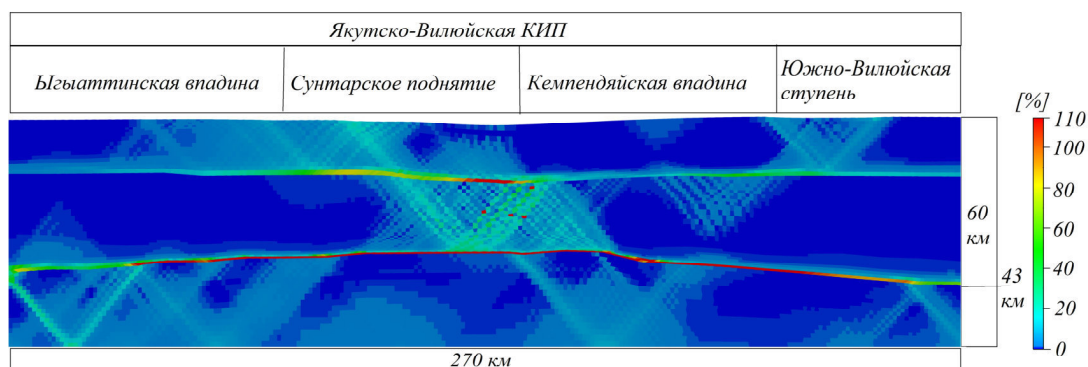
Рис. 2. Распределение неупругой деформации верхней части литосферы на территории Якутско-Вилюйской КИП на основе геологического профиля «Кимберлит–1981»
