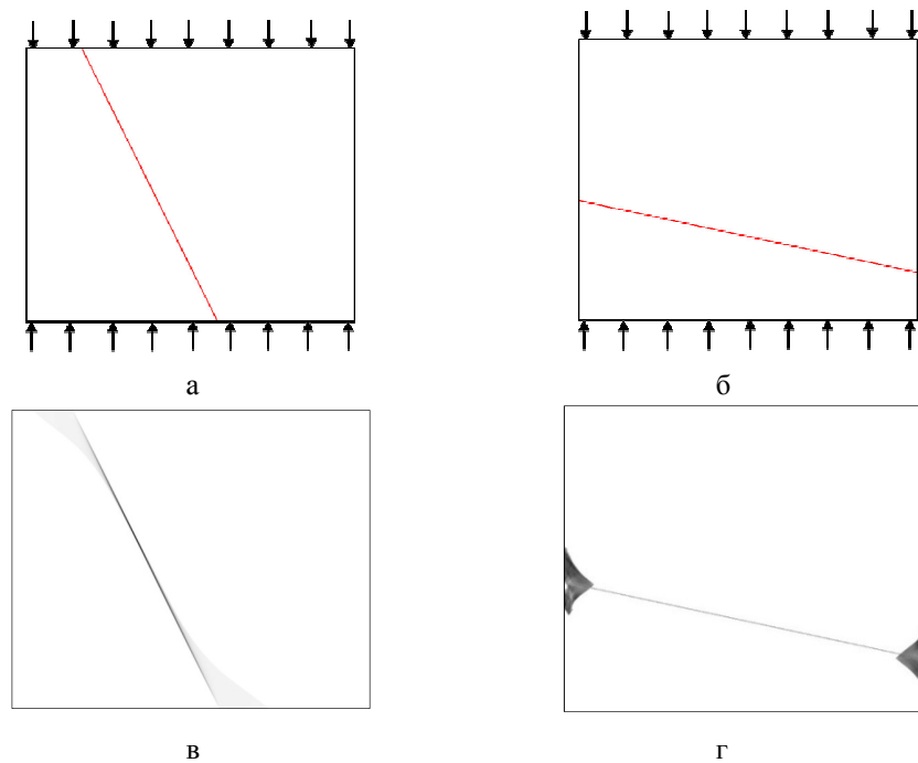
Рис. 1. Модельные карты сред с условиями нагружения и разломами, имеющими разные углы с осью нагружения (а – острый, б – тупой), распространение деформационных фронтов в среде (в, з)
