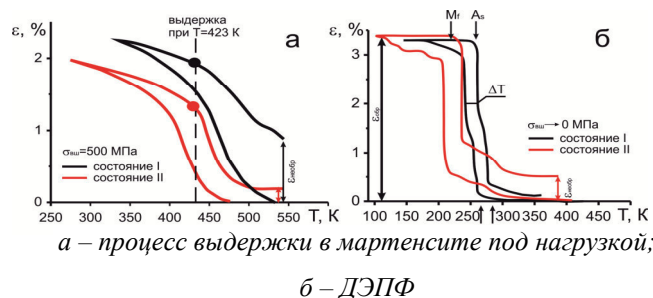
Рис. 1. Кривые \epsilon(T) для монокристаллов Co_{35}Ni_{35}Al_{30}
