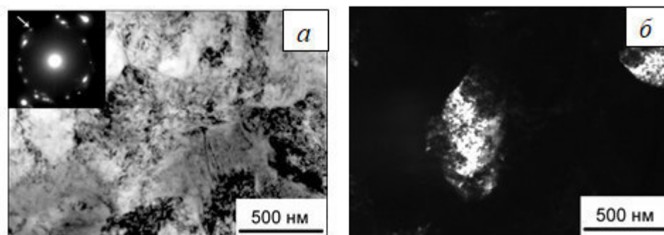
Рис. 1. Типичное электронно-микроскопическое изображение микроструктуры сплава ВТ16: а – светлопольное изображение; б – темнопольное изображение
