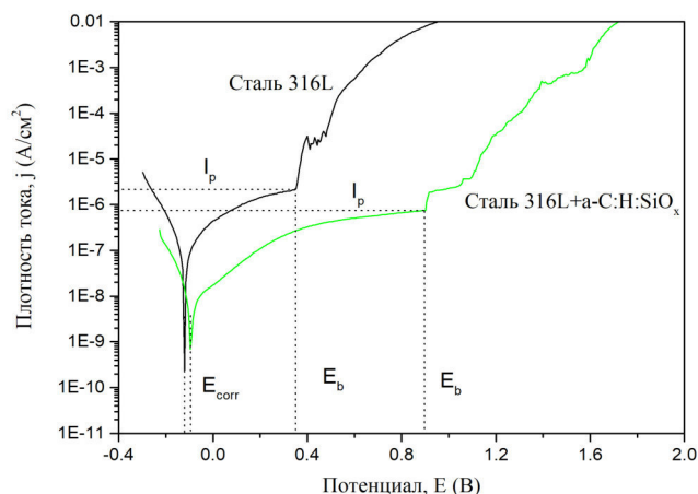
Рис. 1. Поляризационные кривые исходного образца стали AISI 316L и образца стали с нанесенной a\text{-C:H:SiO}_x пленкой в растворе 0.5M NaCl при комнатной температуре
