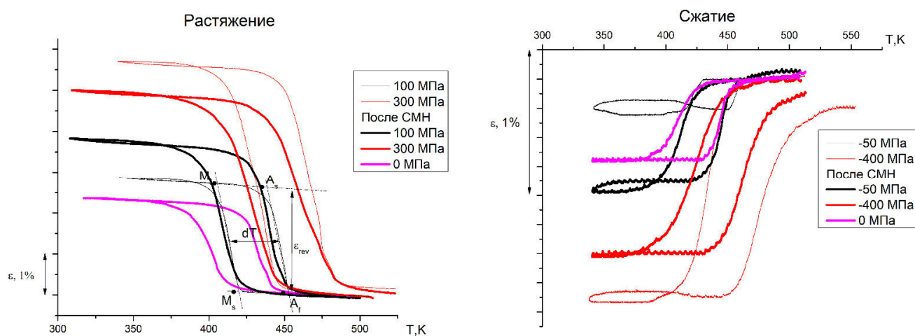
Рис. 1. Кривые \varepsilon(T) для состаренных при 773 К, 3 ч поликристаллов сплава Ni_{50.3}Ti_{32.2}Hf_{17.5} (ат. %) после дополнительного СМН при растяжении и сжатии
