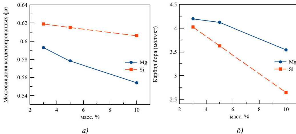
Рис. 2. Зависимость массовой доли конденсированных фаз (а), содержания карбида бора (б) от содержания магния и кремния в смеси
