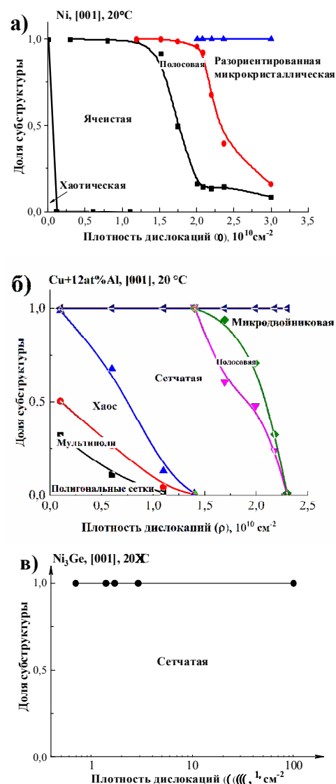
Рис.1. Зависимость долей субструктур деформации монокристаллов чистого Ni (а), монокристаллов твердого раствора Cu-12%Al (б), монокристаллов сплава Ni 3 Ge (в) с ориентировкой оси сжатия [001] от средней скалярной плотности дислокаций
