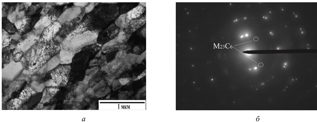
Рис. 2. Микроструктура стали ЭП-823 вблизи области шейки при T=650 °С: а – светлпольное изображение; б – соответствующая микродифракционная картина
