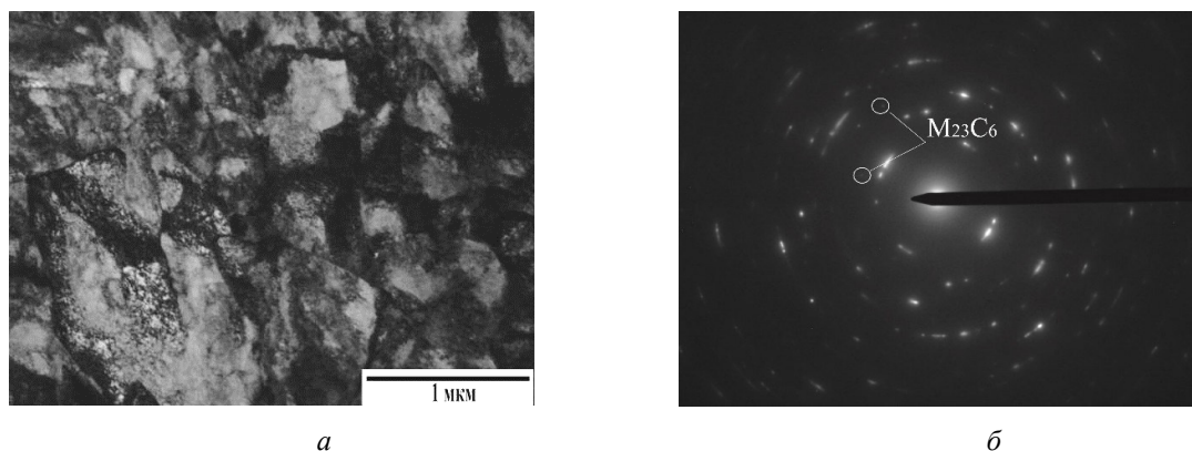
Рис. 1. Микроструктура стали ЭП-823 вблизи области шейки при T = -70 \text{ }^\circ\text{C} : а – светлопольное изображение; б – соответствующая микродифракционная картина
