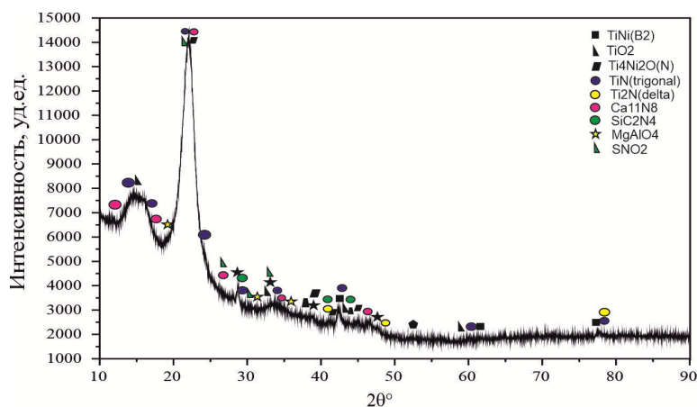
Рис. 2. Рентгеноструктурный анализ пористого СВС- TiNi сплава
