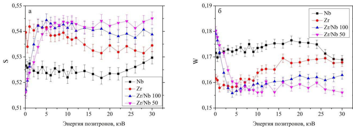
Рис. 1. График зависимости S параметра (а) и W параметра (б) от энергии позитронов НМП Zr/Nb с толщиной индивидуальных слоев 100 \pm 10 нм и 50 \pm 5 нм, а также монослойных покрытий Zr и Nb
