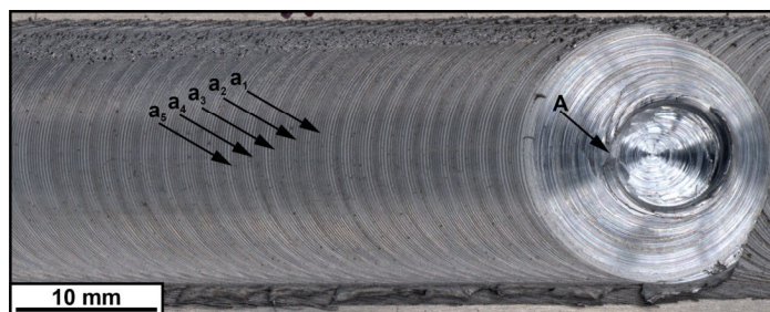
Рис. 3. Строение зоны перемешивания образцов после обработки инструментом с пином квадратного сечения
