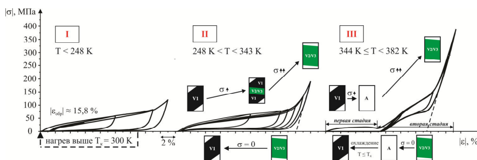
Рис. 2. Кривые \sigma(\varepsilon) для [001]_{B2} -монокристаллов Ni_{49}Fe_{18}Ga_{27}Co_6 в различных температурных интервалах после СМН, полученные в циклах нагрузка/разгрузка
