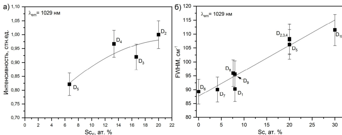
Рис. 2. Зависимость фотолюминесценции от концентрации Sc_Y в додекаэдрической позиции YSAG:Yb (а) и зависимость полуширины основного пика люминесценции от общего содержания Sc в образце (б)
