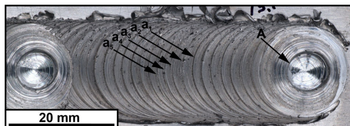
Рис. 2. Строение зоны перемешивания образцов после обработки инструментом с пином квадратного сечения
