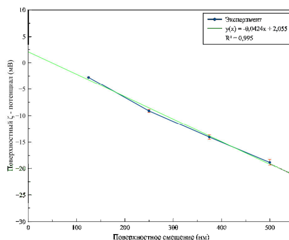
Рис. 1. График значения поверхностного \zeta -потенциала необработанного, спеченного образца Al 2 O 3 с 15% пористостью
