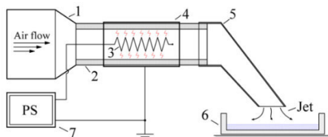
Рис. 1. Функциональная схема лабораторной установки для исследования воздействия на биологические объекты струи плазмы, полученной на основе разряда в потоке воздуха. 1 – компрессор, 2 – кварцевая трубка, 3 – потенциальный электрод, 4 – заземленный электрод, 5 – сопло (силикон), 6 – чашка Петри с обрабатываемой средой, 7 – высоковольтный источник питания
