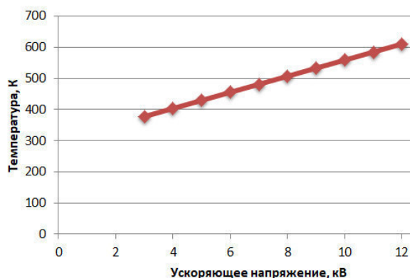
Рис. 3. График зависимости температуры от ускоряющего напряжения
