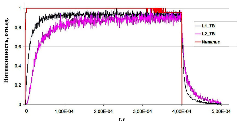
Рис. 1. Нормированные кривые разгорания и затухания электролюминесценции образцов OLED при подаче на них импульсов положительного напряжения прямоугольной формы величиной U=7\text{ В} с длительностью 400\ \mu\text{s} и частотой следования 1\ \text{kHz}
