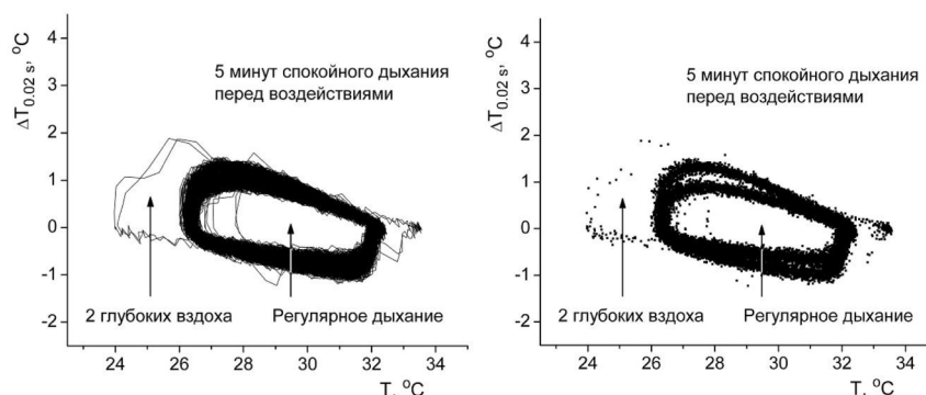
Рис. 1. Фазовая диаграмма дыхания анестезированной крысы в отсутствии внешних интервентных воздействий на организм, построенная по тепловизионному сигналу, измеренному на адсорбционном индикаторе, и отражающая приращение температуры индикатора \Delta T каждые 0.02 с в зависимости от величины этой температуры T . Меньшие значения T соответствуют фазе вдоха, большие – фазе выдоха. Справа – диаграмма, аналогичная левой, представленная в виде экспериментальных точек и выявляющая двухмодовый характер периодического процесса (два «кольца»).
