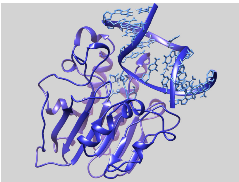
Рис. 1. Общий вид комплекса фермента zApe с ДНК-дуплексом, содержащим AP-сайт
