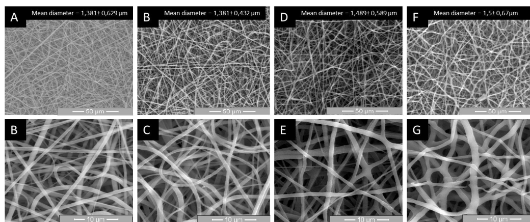
Рис. 1. СЭМ-изображения нановолокон PCL с концентрацией 8 масс.% (A, B ( \times 1000 ), C ( \times 20000 )), 16 масс.% (D, E), 32 масс.% (F, G) парацетамола (от массы сухого полимера) и контрольного образца (A, B)
