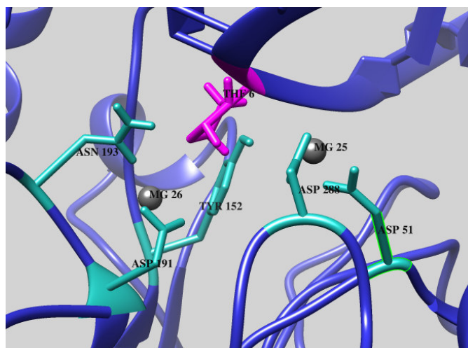
Рис. 2. Схема взаимодействия остатка тетрагидрофурана с аминокислотными остатками zAre и координирующими их двумя ионами магния
