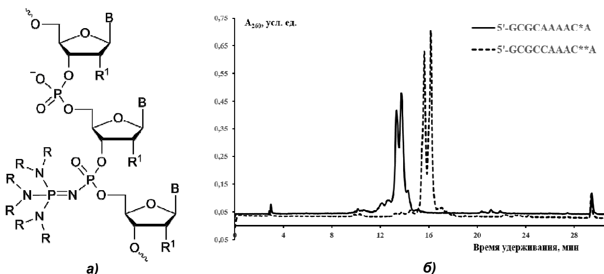
Рис. 1. а) Структура олигонуклеотида с фосфорилфосфазеновой группой, R = \text{Me} , -(\text{CH}_2)_4 , R^1 = \text{H} , \text{OMe} . б) Профили элюции офВЭЖХ олиго-2'-О-метилрибонуклеотидов с фосфорилфосфазеновыми группами, (*) R = \text{Me} , (**) R = -(\text{CH}_2)_4
